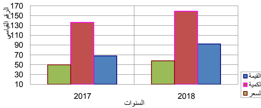
شكل (3) الأرقام القياسية للصادرات النفطية للسنتين (2017-2018) بأساس 2012
