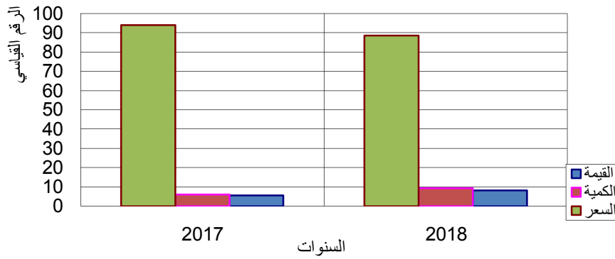
شكل (2) الأرقام القياسية للصادرات غير النفطية للسنتين (2017-2018) بأساس 2012
