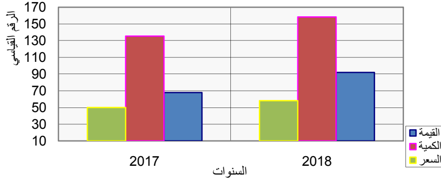
شكل (1) الأرقام القياسية لإجمالي الصادرات للسنتين (2017-2018) بأساس 2012
